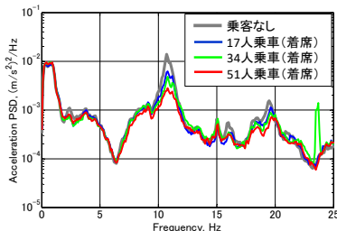
(a) 乗客人数による車体振動の変化
