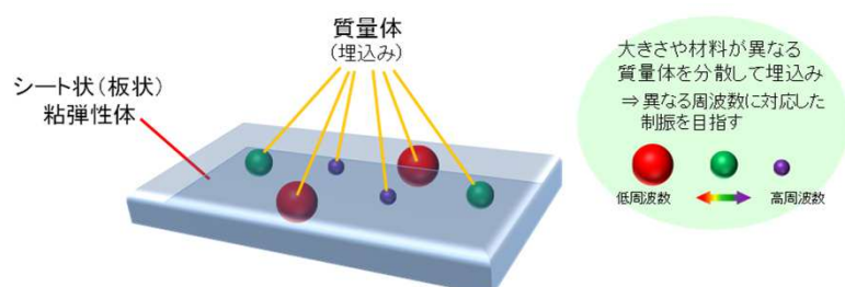
図6 シート状(板状)粘弾性体に埋め込まれた質量体による制振デバイス
