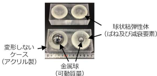
図5 球状粘弾性体で保持された金属球による制振装置 (3)
